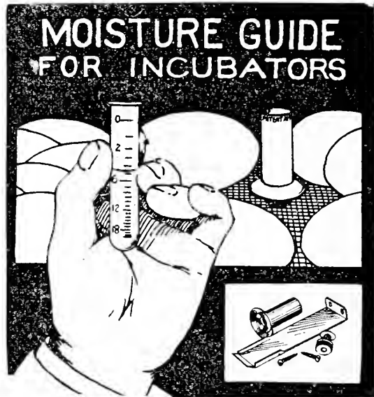
Patterson & Young Moisture Guide
